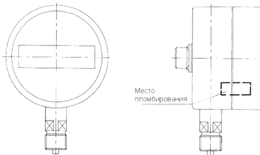
Рисунок 2 - Схема пломбирования от несанкционированного доступа внутрь прибора DM5002M
